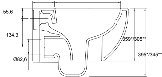
SEZIONE A-A
