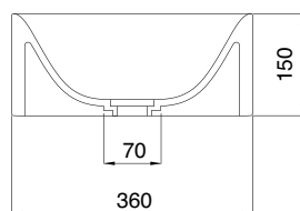
SEZIONE A-A
