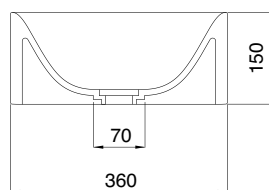
SEZIONE A-A
